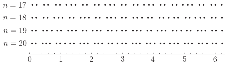
Slika 3.1: Nule ortogonalnog trigonometrijskog polinoma polu-celobrojnog stepena A_{n+1/2}^C u odnosu na težinsku funkciju w(x) = 1 + \sin 15x , x \in [0, 2\pi) , za n = 17(1)20
