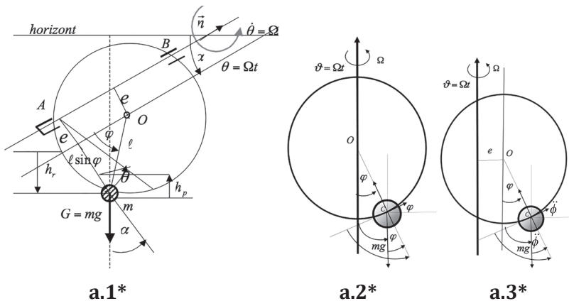
Слика 9. a* Модели тешке материјалне тачке која се креће по ротирајућем кругу, константном угаоном брзином, око ексцентричне осе косо постављене у односу на хоризонт ( a*1 ), односно вертикалне центричне ( a*2 ) или вертикалне ексцентричне осе ( a*3 ).
