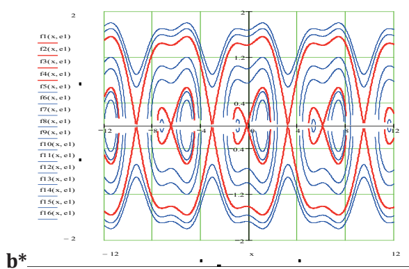
Слика 9. b* Фазни портрет нелинеарне динамике тешке материјалне тачке креће се по ротирајућем кругу, константном угаоном брзином, око ексцентричне вертикалне осе, приказане на слици ( a*3 ).
