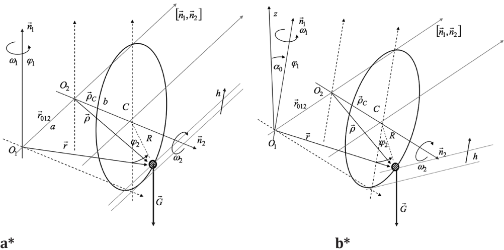
Слика 11. Кретање тешке материјалне тачке спрегнутим ротацијама око ортогоналних мимоилазних оса, од којих је фиксирана оса вертикална ( a* ), односно коса у односу на вертикалу ( b* ).
