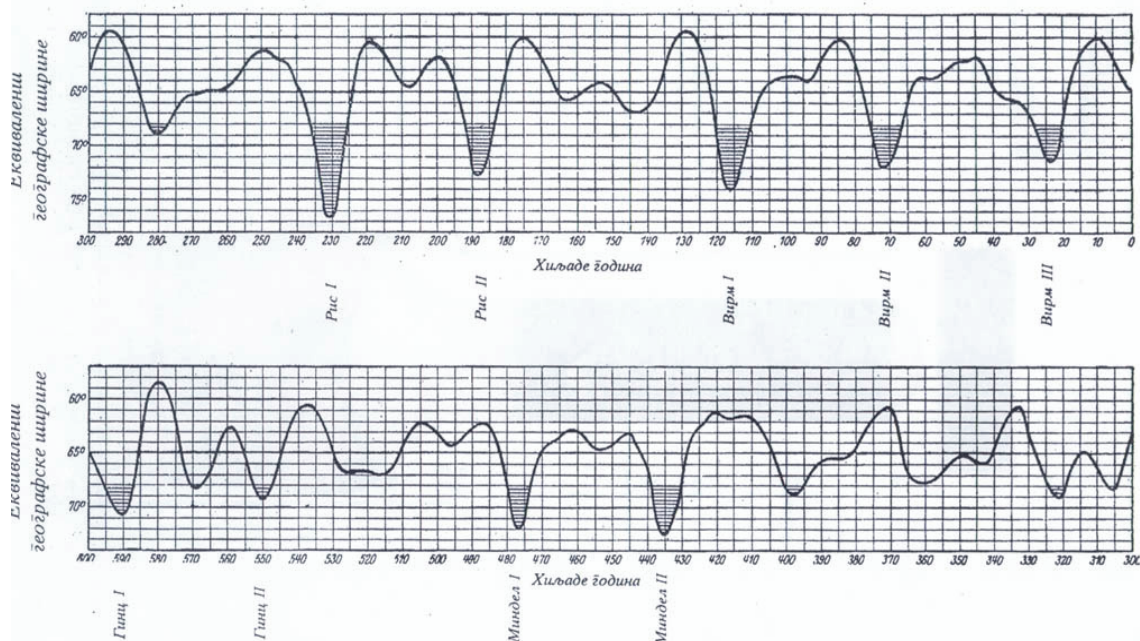
Слика 10. Миланковићева крива осунчавања. На апсциси је време од данашњег тренутка обележеног са 0 до 600.000 година уназад, а на ординати је еквивалентна ширина која показује којој данашњој географској ширини одговара осунчавање на ширини 65^\circ у неком тренутку прошлости.
